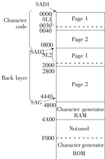
图 3 RA8835 的内存地址划分
