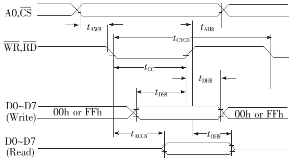
图 2 RA8835 读写时序图
