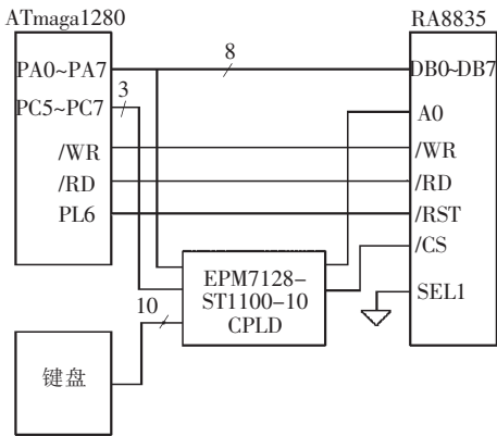
图 1 ATmega1280 与 RA8835 的硬件接线图
